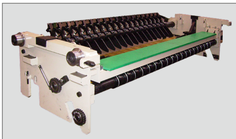
Gruppon arpa di taglio / Harp type cutting unit / Grupo de alambre de corte
